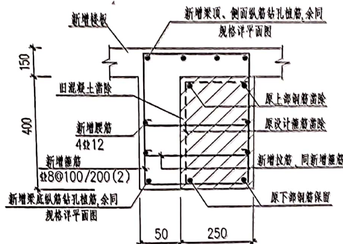
基础梁加固大样
